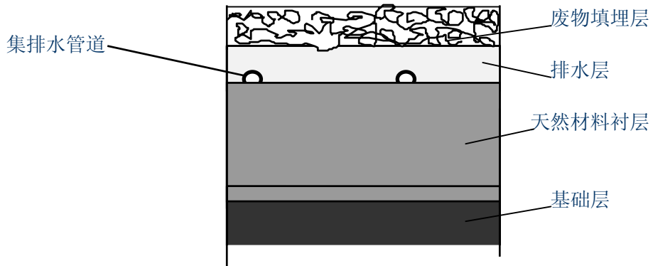
图3 天然材料衬层示意图
