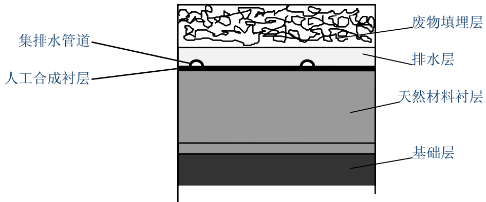
图2 复合衬层示意图
