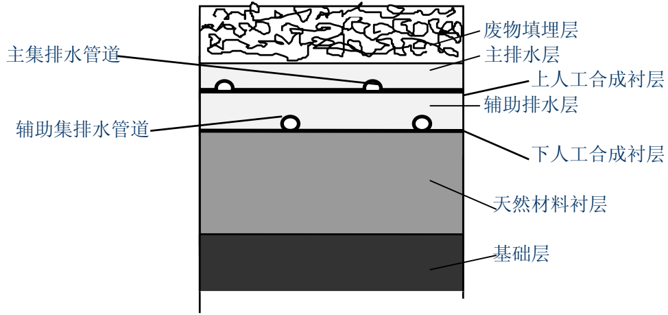
图1 双人工衬层示意图
