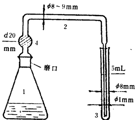
砷化氢发生与吸收装置图
